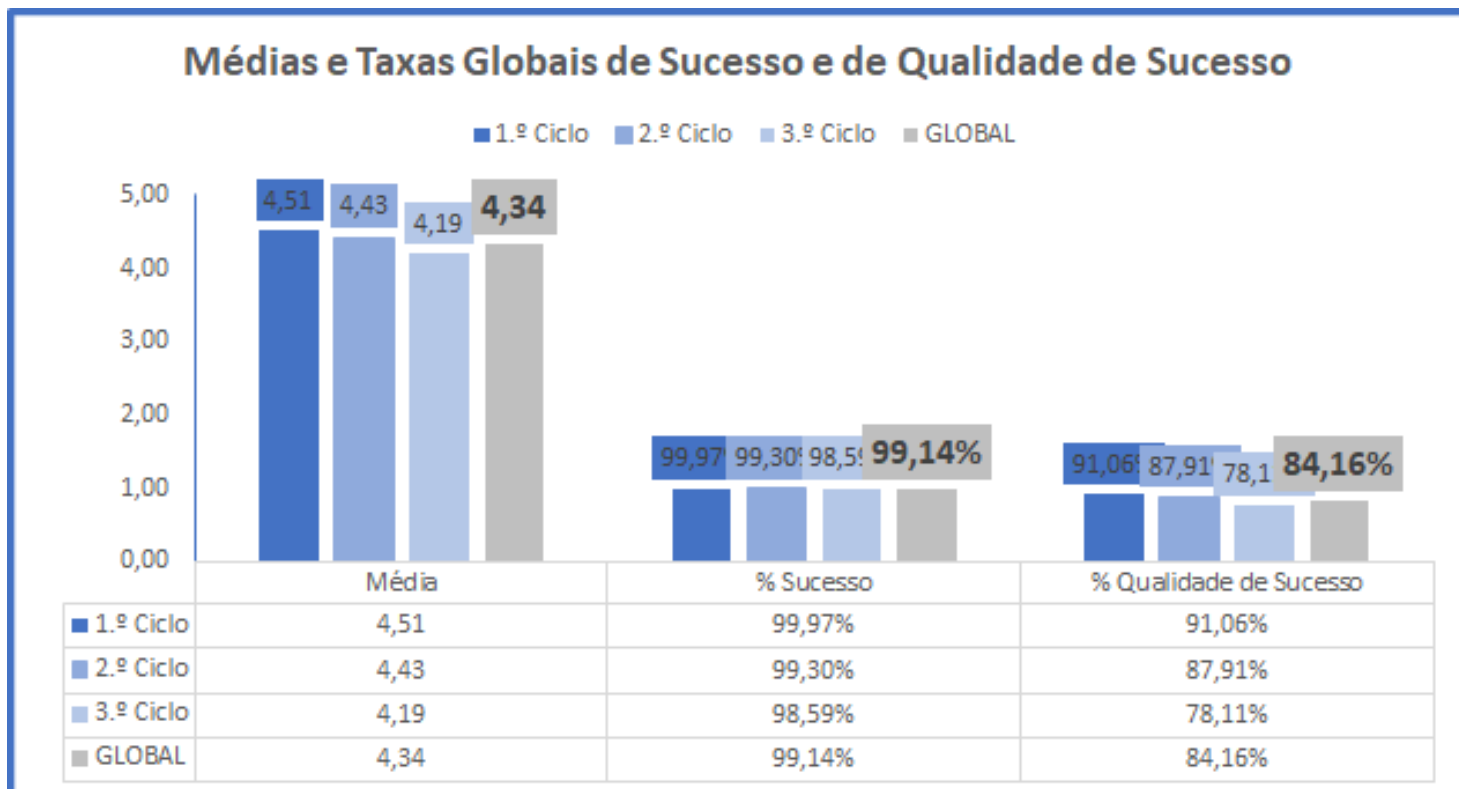
QUADRO 2 - Médias e Taxas Globais de Sucesso e Qualidade de Sucesso
